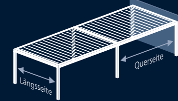
Kopplung in Querrichtung (Anlagen voreinander an der Wand) max. 24 Meter
